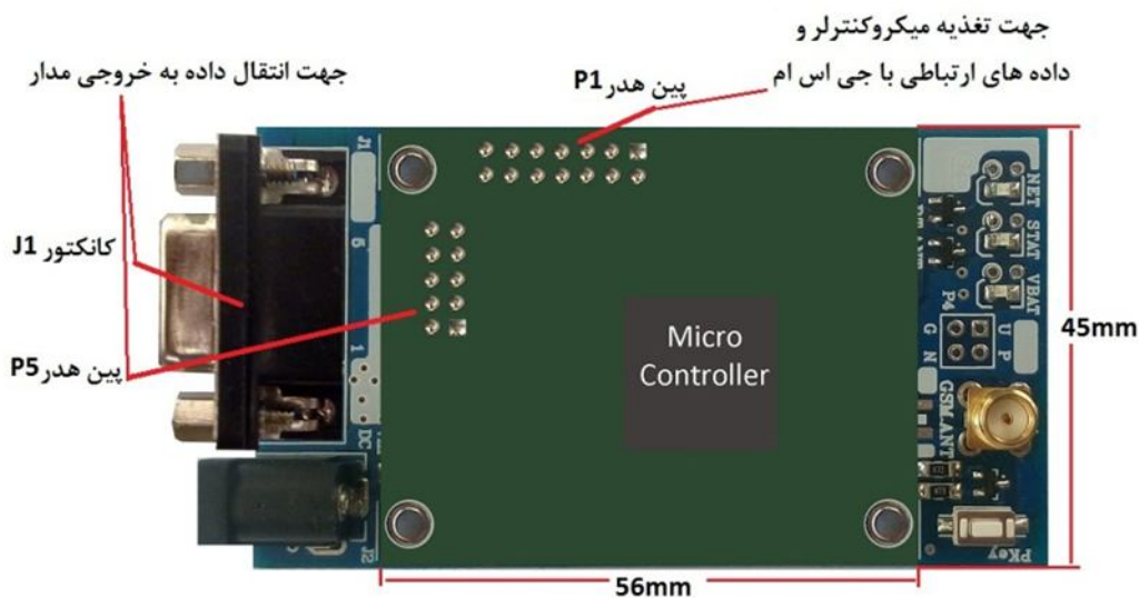
شکل 6: طراحی و نصب برد کنترل
