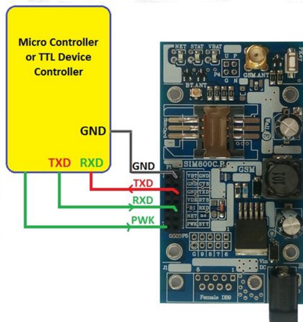
شکل 5: اتصال برد توسعه ABg144P-C به میکروکنترلر
