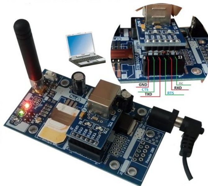
شکل 2: اتصال برد توسعه ABg144P-C به رایانه توسط مبدل یو اس بی
