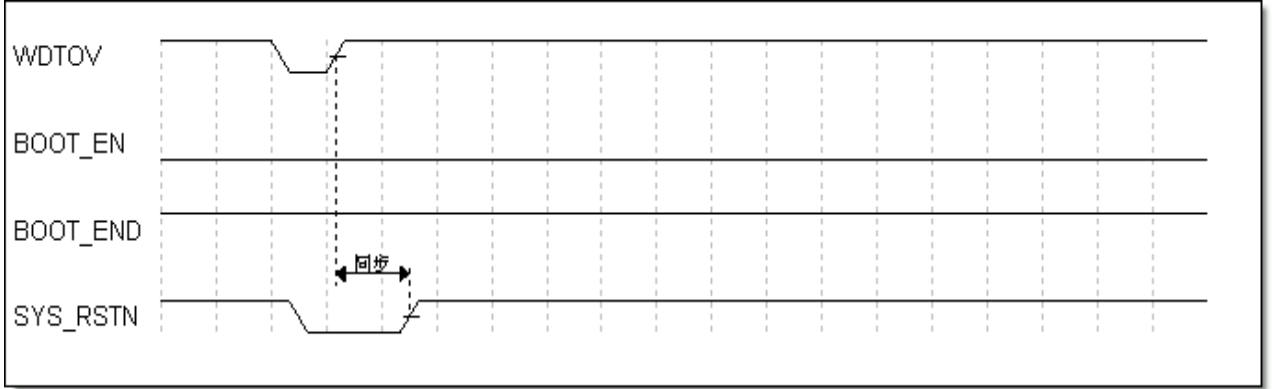
图 4.5 WDT 复位不产生 BOOT
