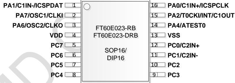
图 1.6 SOP16
