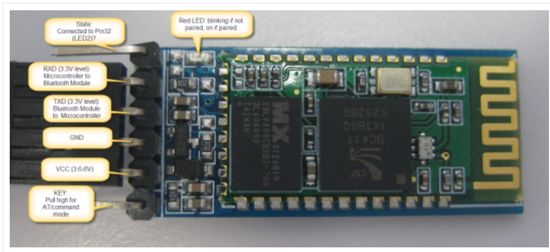
— HC-06 Top Side
