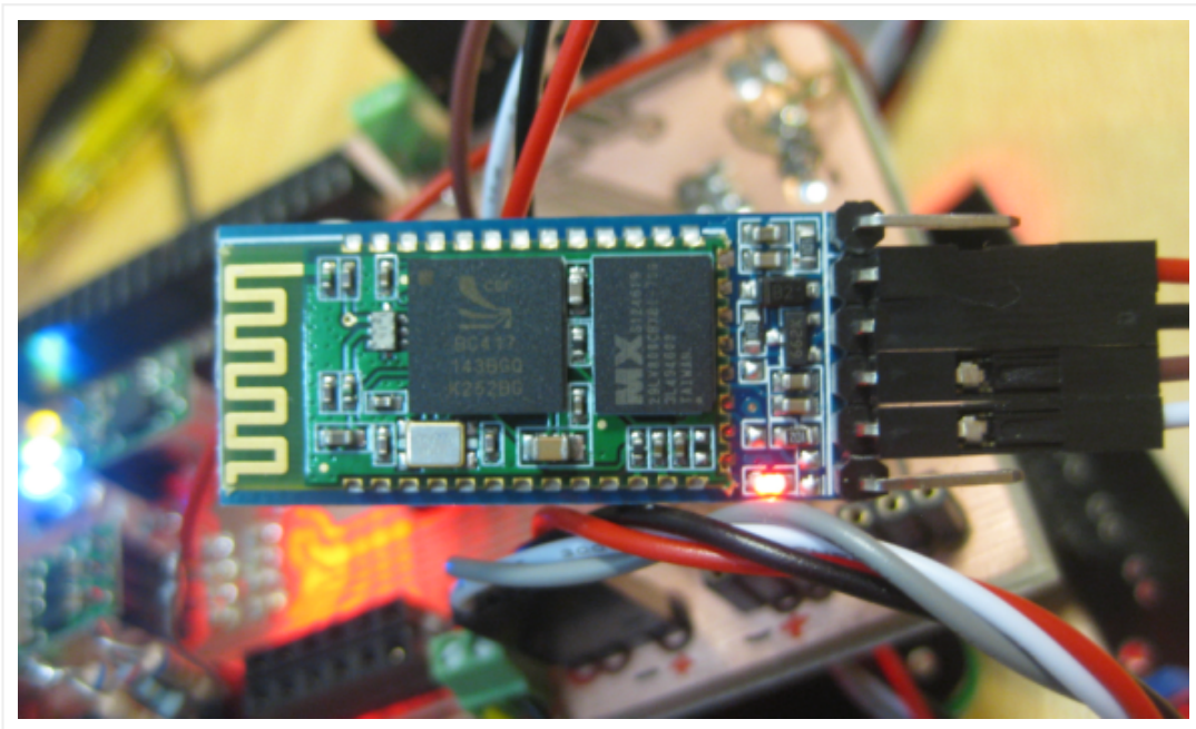
— DX.com Bluetooth Module (HC-06)
