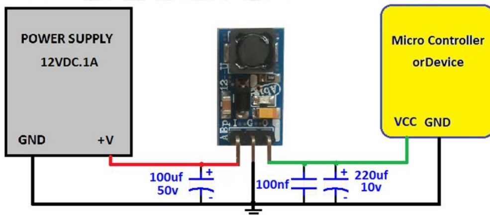
شکل 1: راه اندازی و اتصال خازنهای خارجی مبدل ABp123CU
