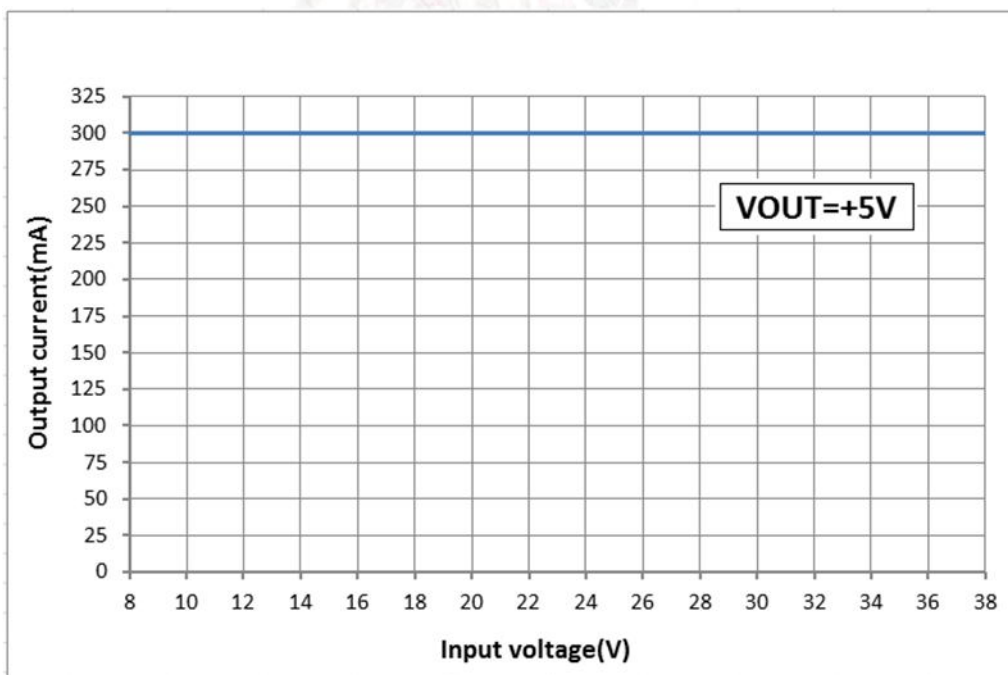
8. نمودار ولتاژ - جریان مبدل ABp123CU
