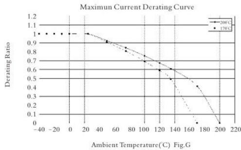
Ambient Temperature(°C) Fig.G
