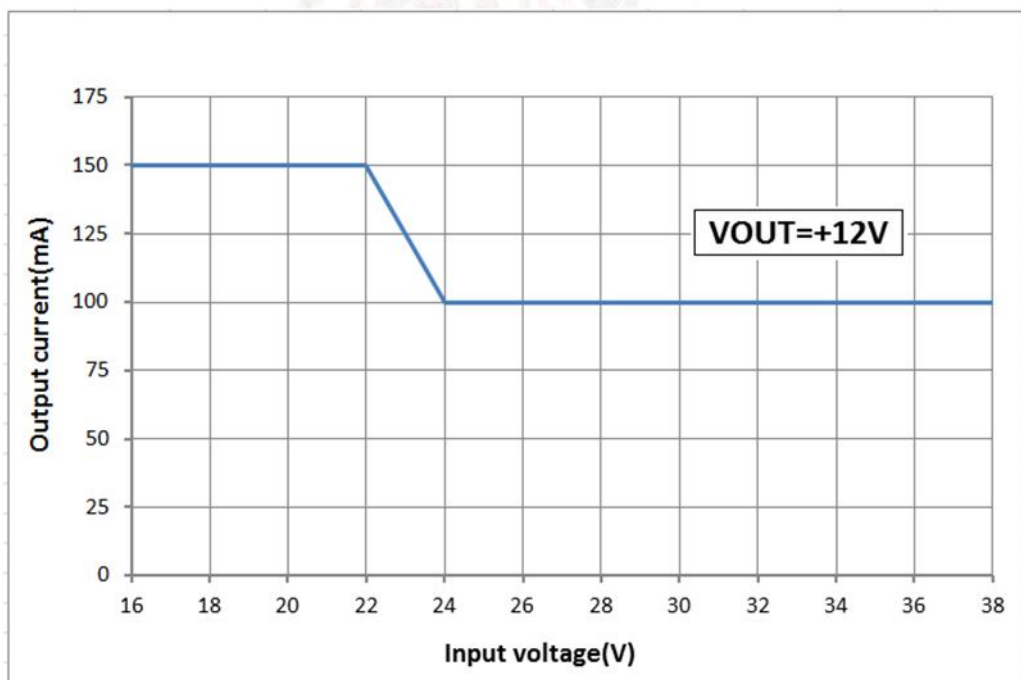
8. نمودار ولتاژ - جریان مبدل ABp124CU
