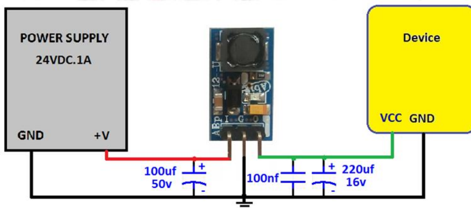
شکل 1: راه اندازی و اتصال خازنهای خارجی مبدل ABp124CU
