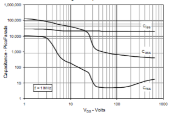
Fig. 12. Capacitance
