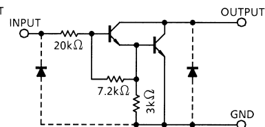
TD62105P / F
