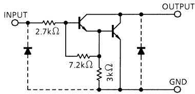
TD62103P / F
