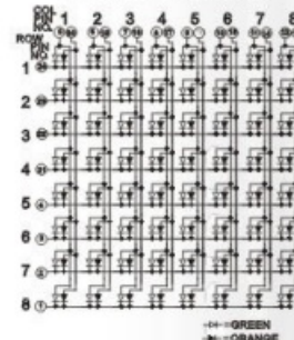
PCB:M15088C/DEG
