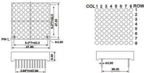
CPM19088
