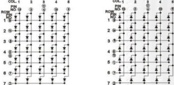
PCB:M20057A/B
