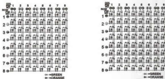
PCB:M19088A/BEG
