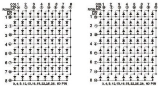
PCB:M19088A/B
