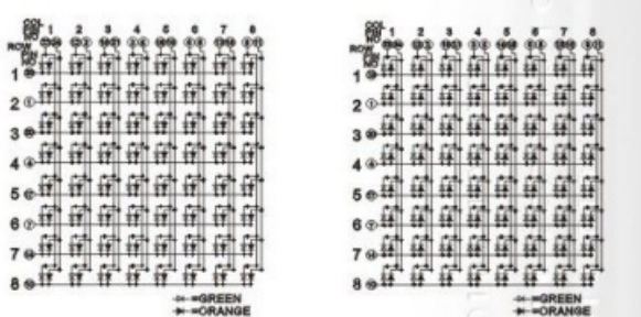
PCB:M19088C/DEG
