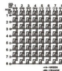
PCB:M12088AB/E
