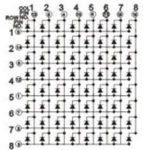
PCB:M15088A/B
