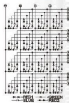
PCB:M15088A/BRGB
