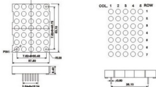
CPM20057
