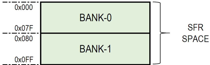
图 15-2 间接寻址
