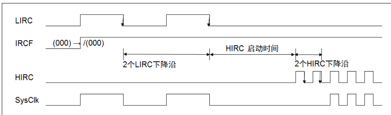
图 6-3 由 LIRC 切换到 HIRC 时序图 (同样的原则也适用于 EC, LIRC, HIRC 之间的切换)
