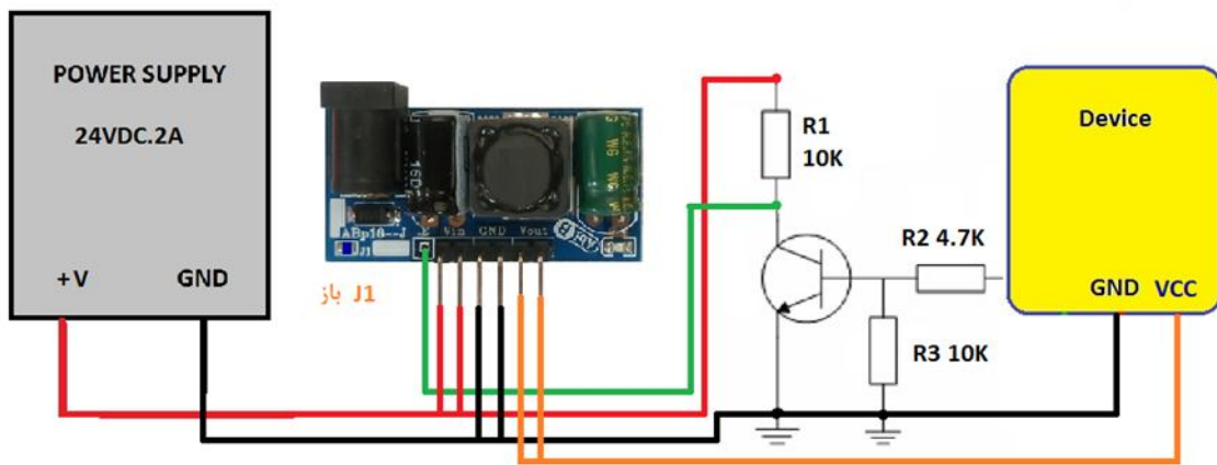
شکل 3: راه اندازی مبدل ABp164BJ-C با پین فعال ساز
