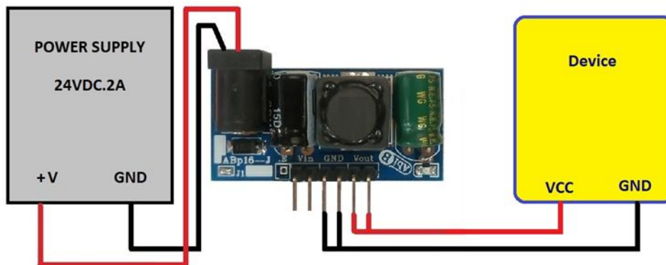
شکل 2: راه اندازی مبدل ABp164BJ-C بدون پین فعال ساز
