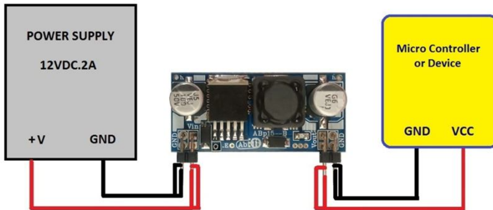
شکل 2: راه اندازی مبدل ABp152BB-C بدون پین فعال ساز
