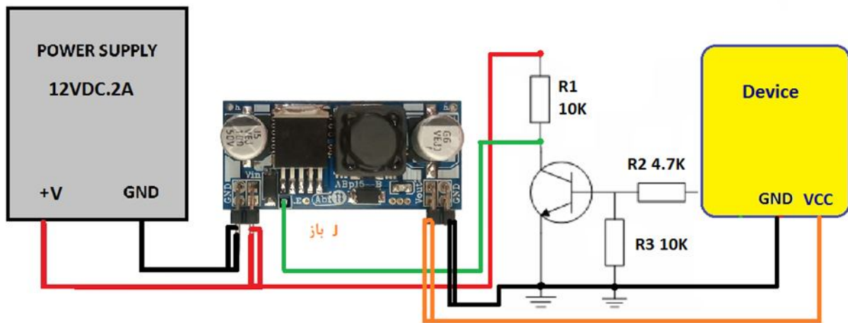
شکل 3: راه اندازی مبدل ABp152BB-C با پین فعال ساز
