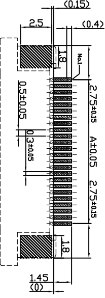
适用线路板 RECOMMENDED PCB LAYOUT
