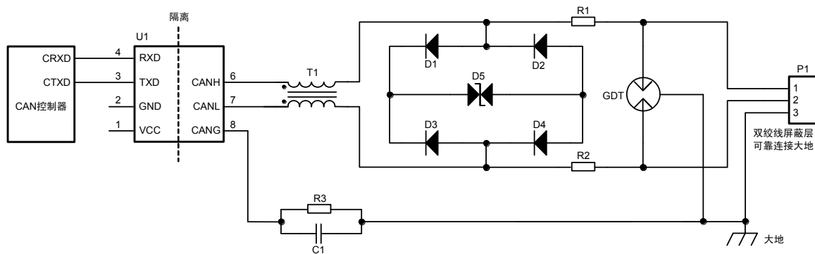
图 3 端口保护推荐电路
