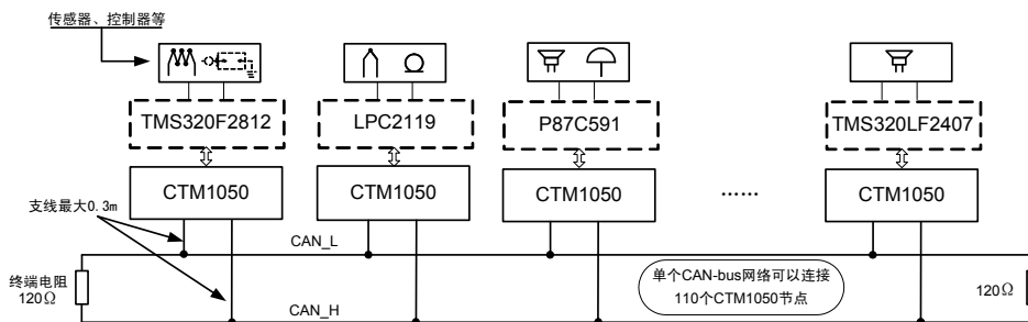
图 2 单个 CAN-bus 典型网络连接示意图
