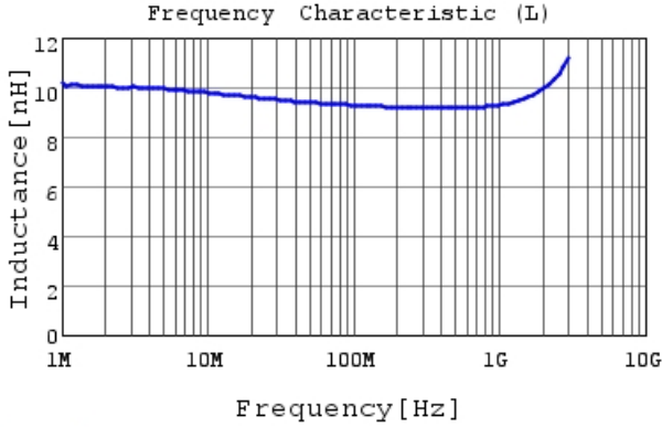
LQW18AN9N1G80 L
