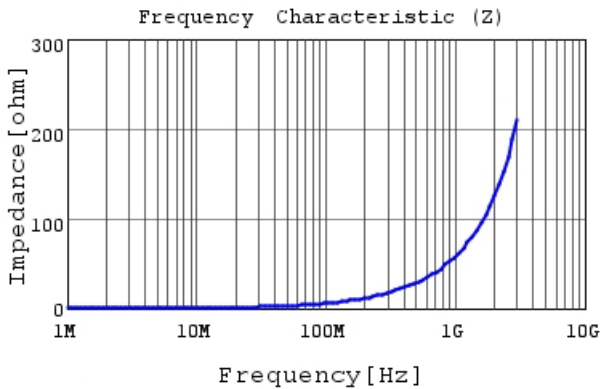
LQW18AN9N1G80 |Z|
