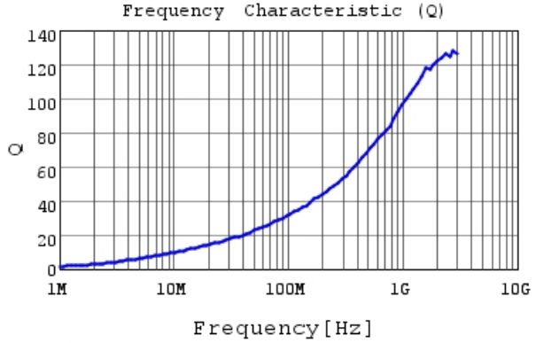
LQW18AN9N1G80 Q
