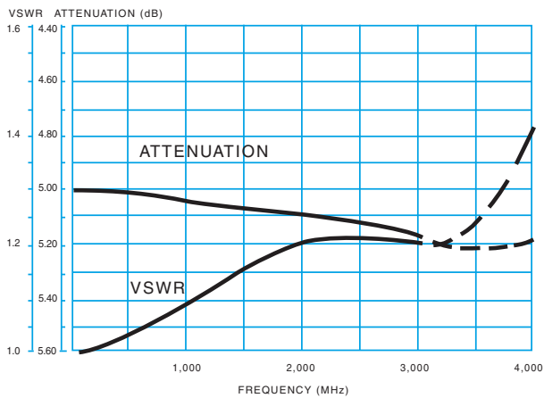
5 dB ATTENUATOR
