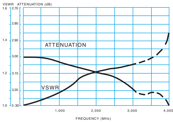
3 dB ATTENUATOR
