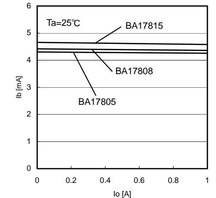
Fig.24 出力電流—バイアス電流
