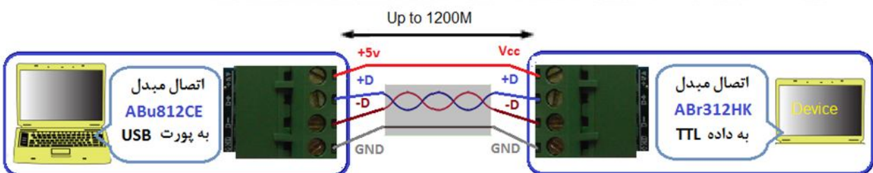
- اتصال Point to Point مبدل به دستگاه سریال RS485 با تامین تغذیه .
