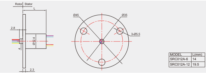
外形尺寸 OUTLINE DIMENSION 单位(UNIT) mm
