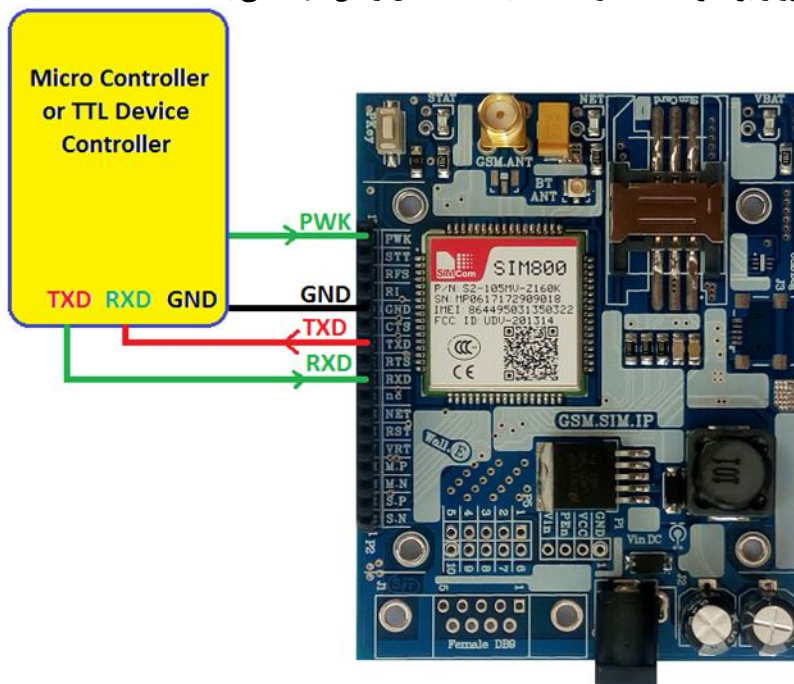
شکل 5: اتصال برد توسعه ABg114N-C به میکروکنترلر
