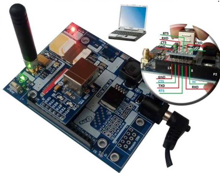
شکل 2: اتصال برد توسعه ABg114N-C به رایانه توسط مبدل یو اس بی
