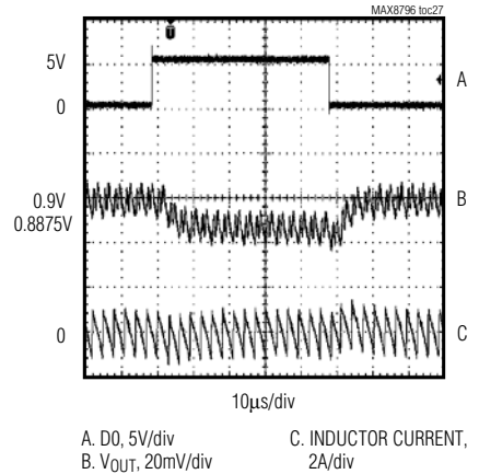
DO 12.5mV DYNAMIC VID CODE CHANGE
